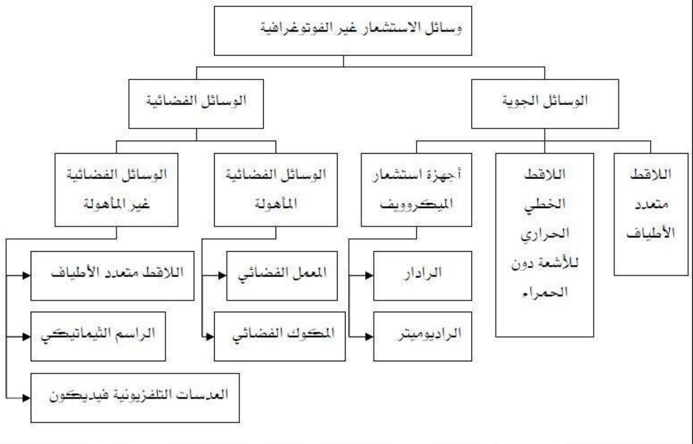
شكل (2 - 6) وسائل الاستشعار غير الفوتوغرافية بحسب وسيلة الحمل
